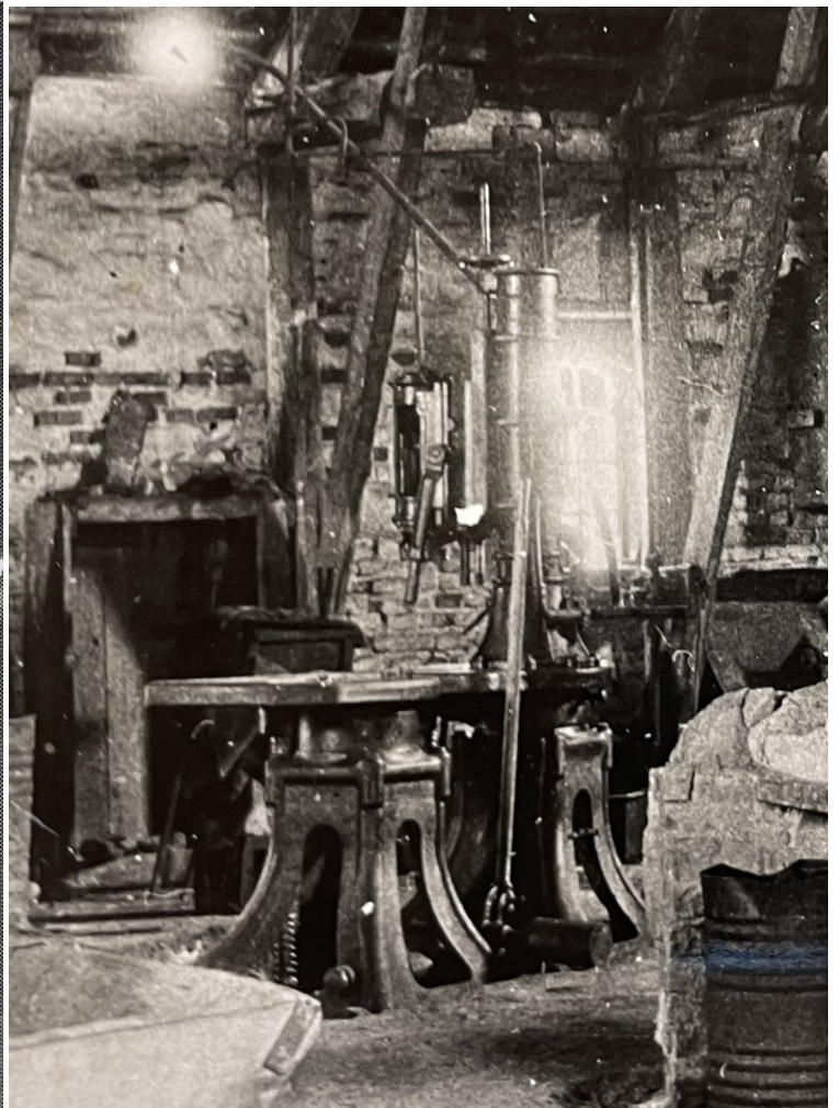
Den Halvautomatisk flaskemaskine af fabrikatet Aftergut
